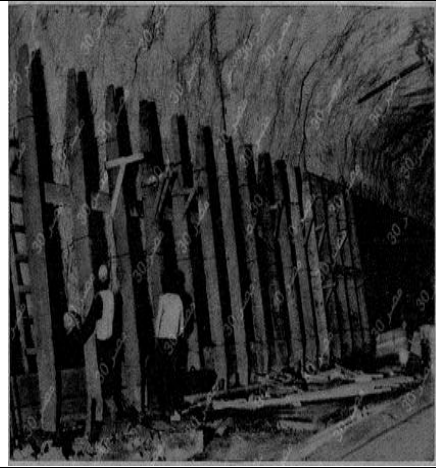
(لوحة ٨) صور توضح عمل البلوكات الخرسانية داخل النفق؛ عن مجلة المصور.
