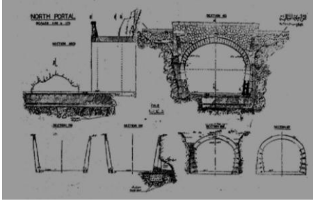
قطاع هندسى يوضح الواجهة الشمالية
